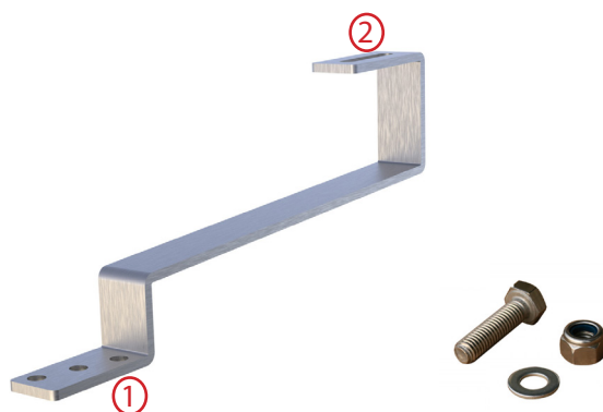
Illustration 1 : Ancrage à la surface de la toiture
